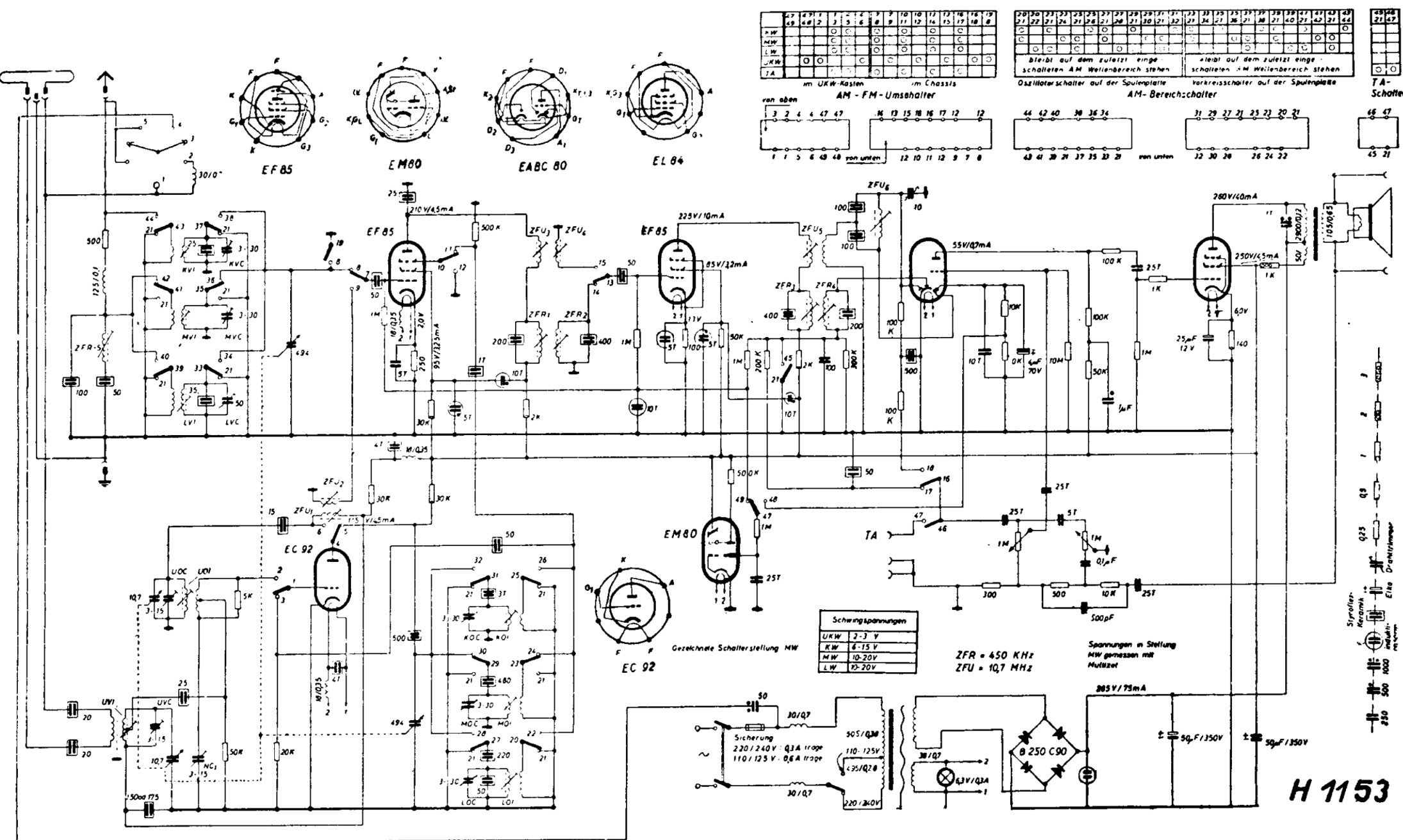
BLAUPUNKT (Blaupunkt Werke GmbH, Hildesheim) - Mod. Roma. Apparecchio AM/FM. Onde lunghe da 160 a 350 kc/s, onde medie da 546 a 1500 kc/s, onde corte da 6,05 a 15,4 Mc/s, onde ultracorte (FM) da 87 a 100 Mc/s. MF/AM a 450 kc/s, MF/FM a 10,7 Mc/s. Sensibilità d'antenna 10 \mu V per OM, 15 \mu V per OL e 20 \mu V per OC. Potenza d'uscita 3 watt indistorti.
